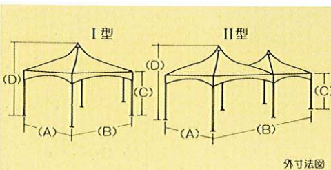
外寸法図
